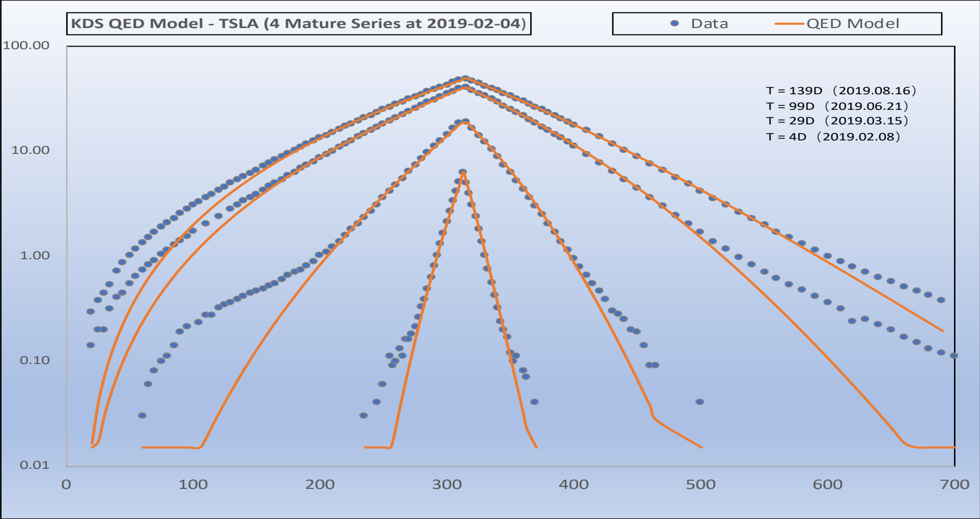
● 该图显示的是交易所交易股票TSLA的外价（OTM）期权价格作为执行价格的函数。实线代表QED模型，圆圈代表期权交易数据。
